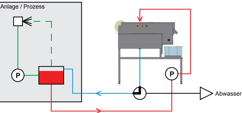
Exécution By-Pass [A10 avec option P + K2]
